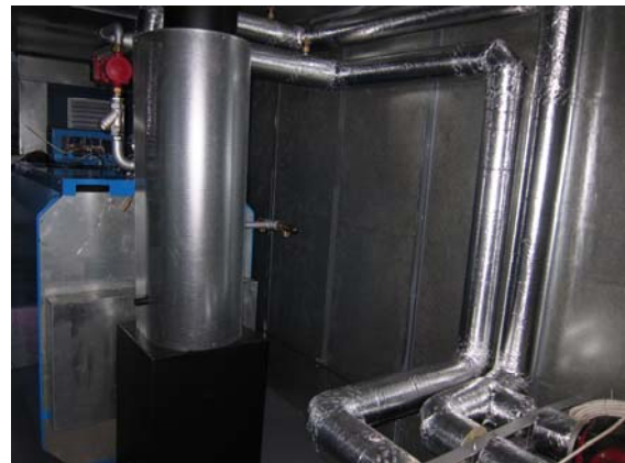
Tur- returrør med shuntpumpe
